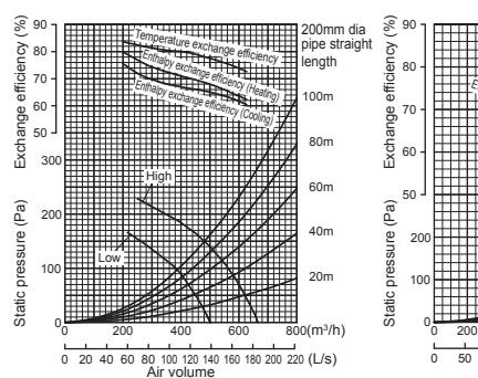
GUF-50RD4
